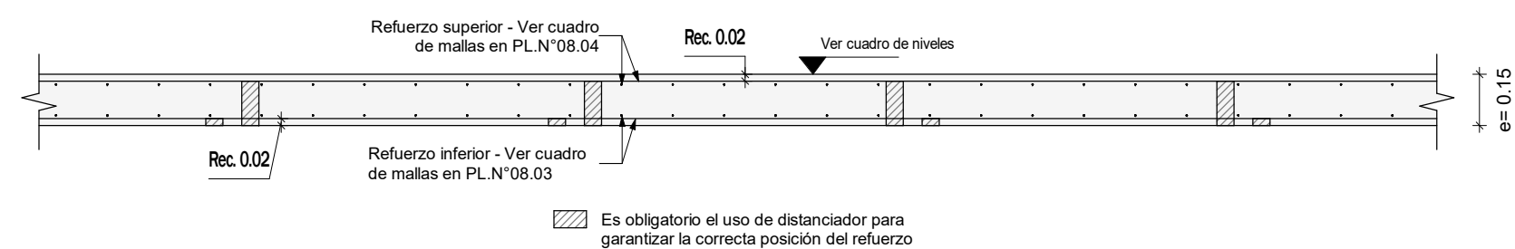
CORTE TÍPICO PLACA ÁEREA e=0.15 Escala 1 : 20
