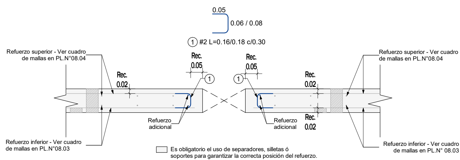
DETALLE TÍPICO - UBICACIÓN REFUERZO ADICIONAL Escala 1 : 10
