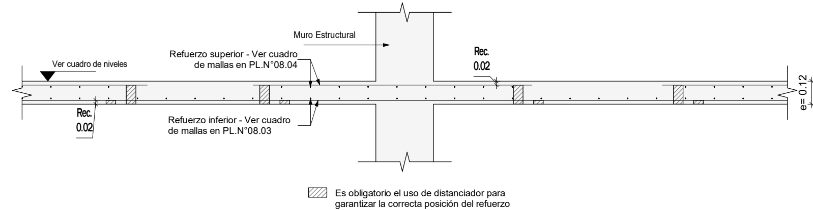
CORTE TÍPICO PLACA ÁEREA e=0.12 Escala 1 : 20
