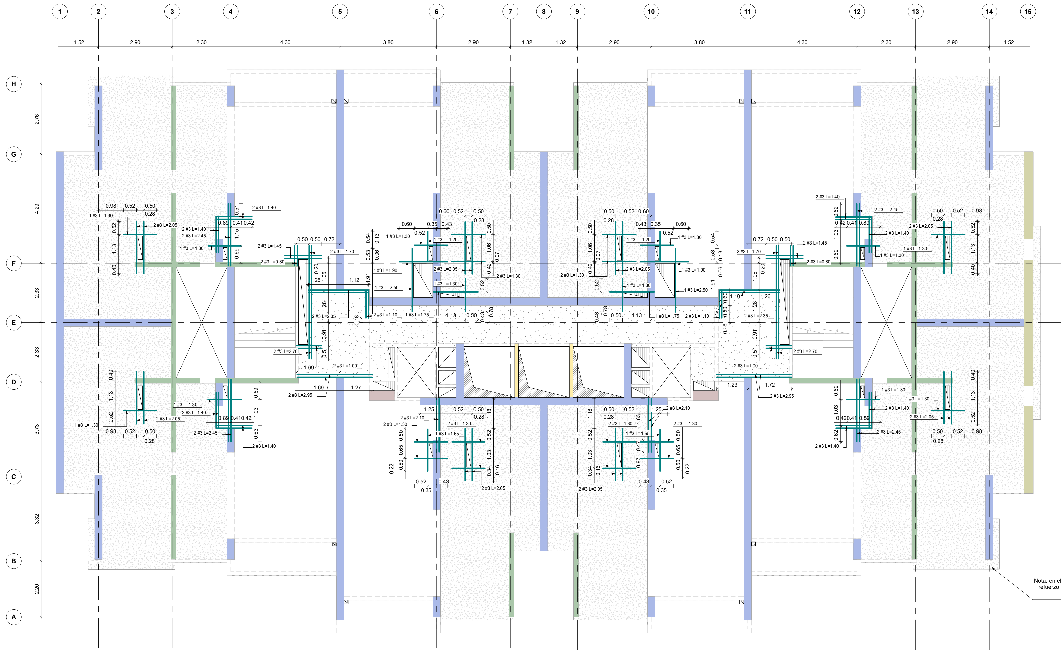
PLANTA DE REFUERZO ADICIONAL PISO TIPO 3 ( PISO 23 A PISO 28 ) Escala 1 : 75
