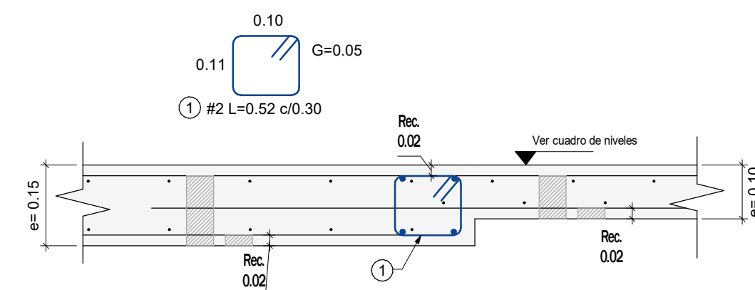
DETALLES TÍPICOS - CAMBIO DE SECCIÓN Escala 1 : 10
