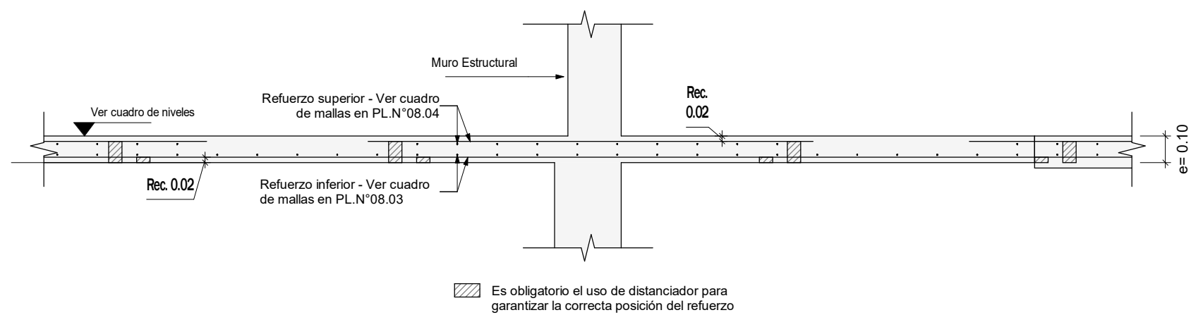
CORTE TÍPICO PLACA ÁEREA e=0.10 Escala 1 : 20
